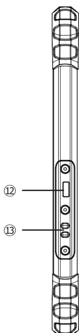
左側面
