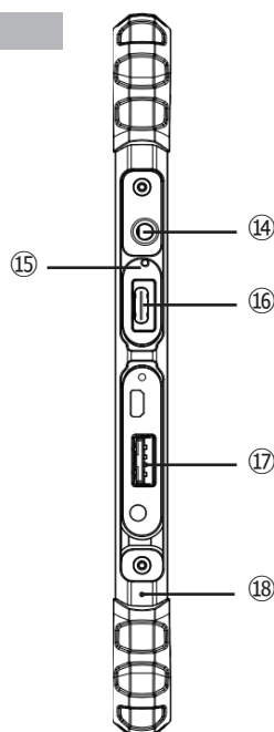
右側面
