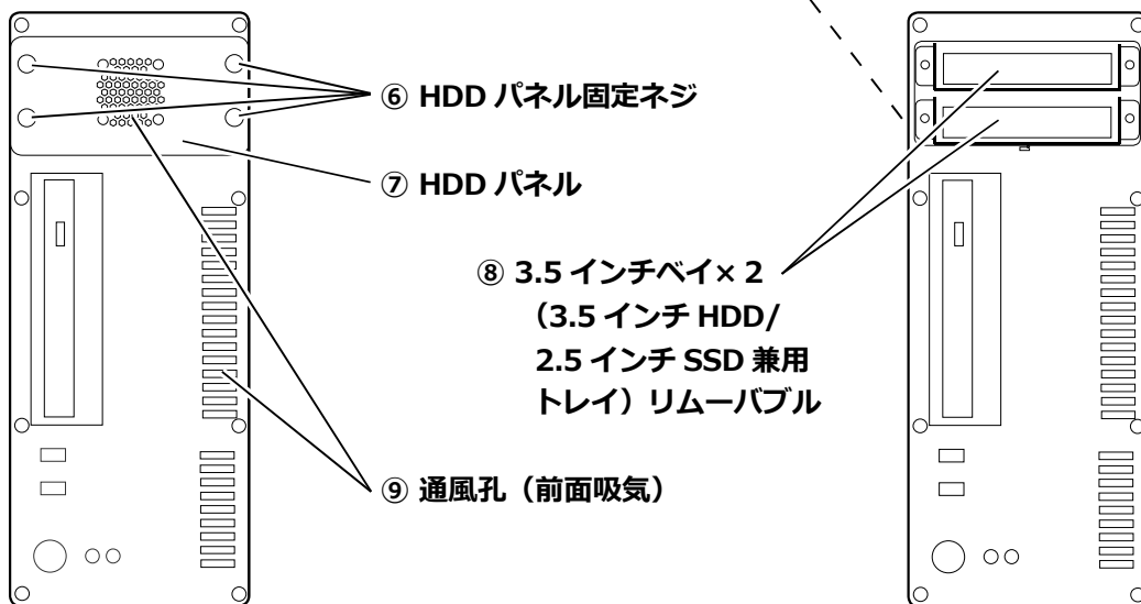
HDD パネルを外した場合
